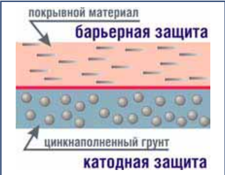
Рис.2 Схема комбинированной системы защитного покрытия на основе цинкнаполненной грунтовки и покрывной эмали
