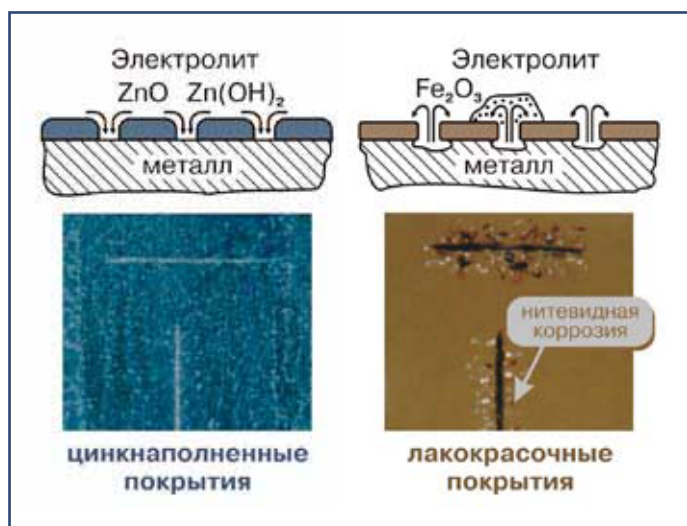
Рис.1 Особенности механизма защитного действия цинкнаполненных (а) и лакокрасочных (б) покрытий. Вверху – схема протекания коррозионных процессов. Внизу – внешний вид покрытий после ускоренных коррозионных испытаний (у лакокрасочного покрытия видна интенсивная нитевидная коррозия вдоль искусственно нанесенных дефектов – надрезов)
